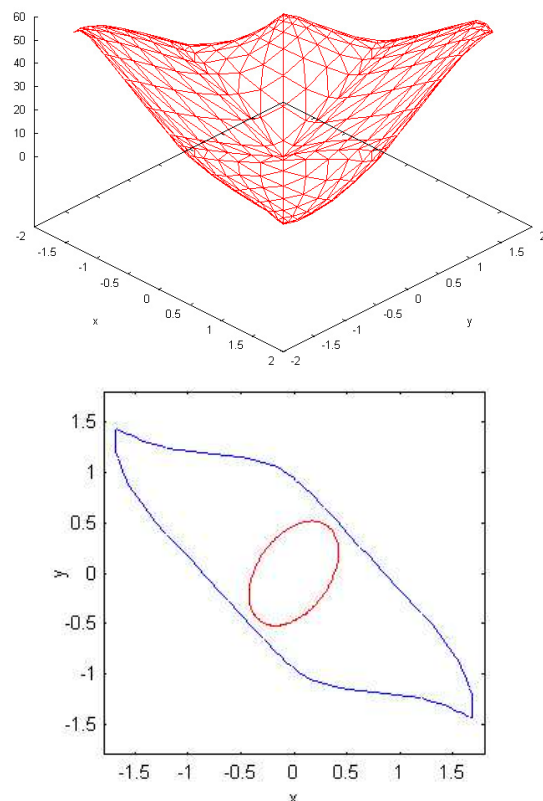
Mynd 2. Að ofan er graf Lyapunov-falls fyrir verkefni (10), stikað út frá lausn viðkomandi bestunarverkefnis, og að neðan er undirmat \mathcal{R}_{Att} .
