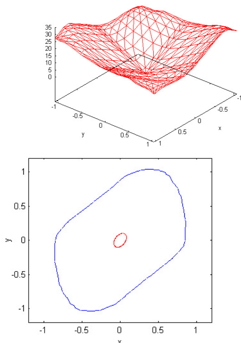
Mynd 1. Að ofan er graf Lyapunov-falls fyrir verkefni (9), stikað út frá lausn viðkomandi bestunarverkefnis, og að neðan er undirmat \mathcal{R}_{Att} .
