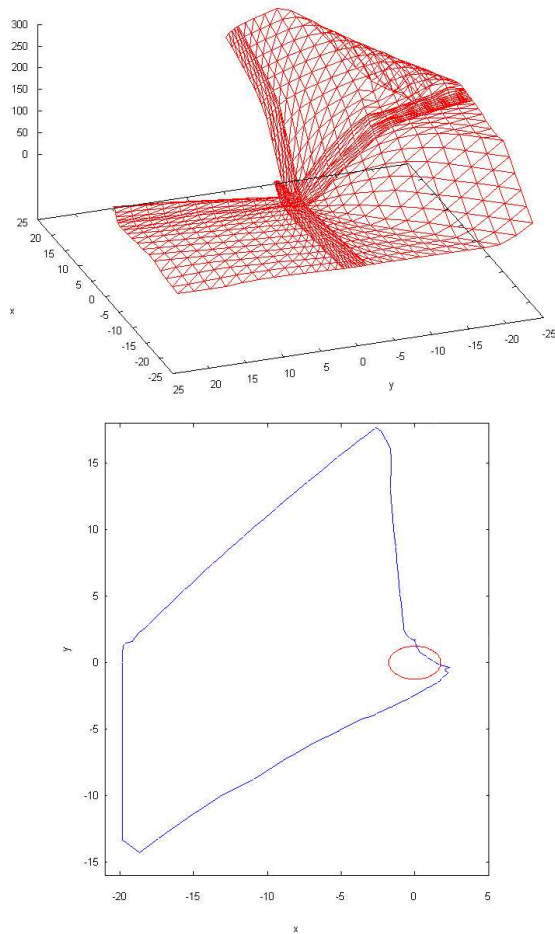
Mynd 3. Að ofan er graf Lyapunov-falls fyrir verkefni (11), stikað út frá lausn viðkomandi bestunarverkefnis, og að neðan er undirmat \mathcal{R}_{Att} .
