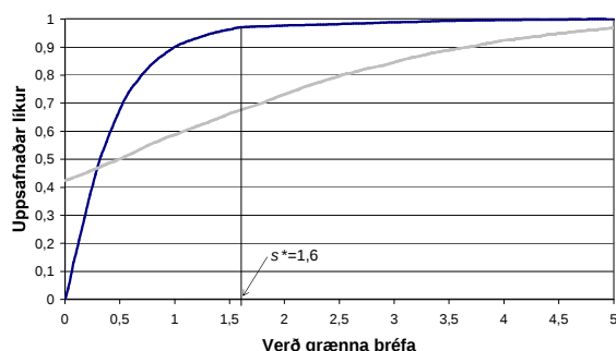
Mynd 3. Uppsafnað dreififall fyrir hermd gildi á verði grænna bréfa. Ferillinn sem byrjar í 0 sýnir verð með flutningi milli tímabila, en hinn sýnir verð án flutnings milli tímabila
